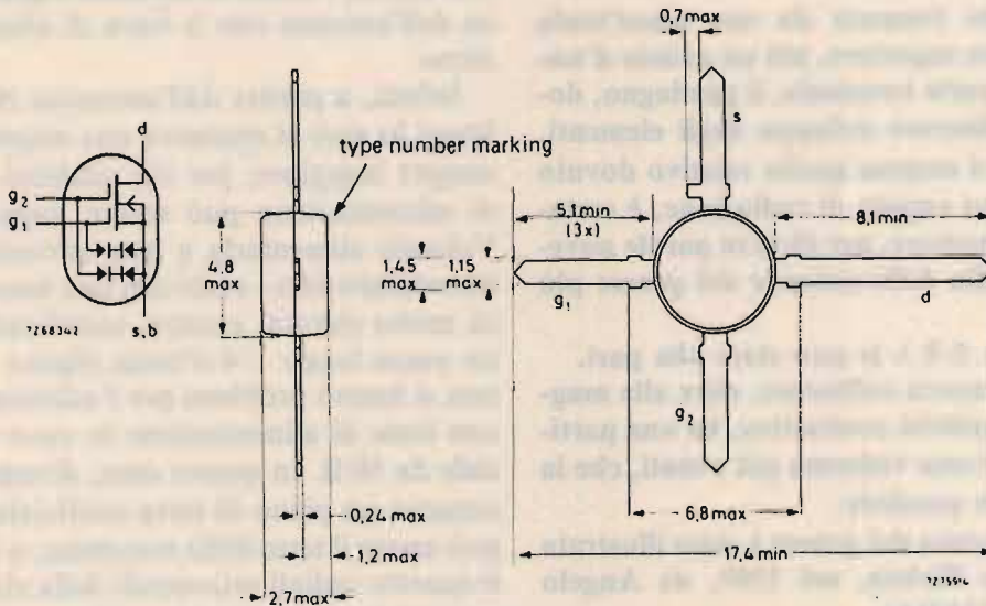
Fig. 1 SOT-103.
